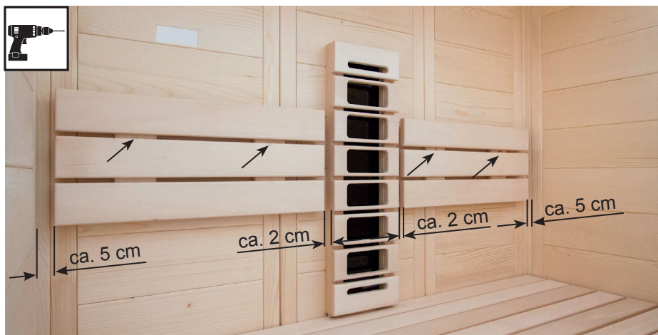
Punta per trapano da 3 mm, 4 viti 4 x 70 mm
