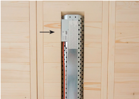
Anschlussbox oben
