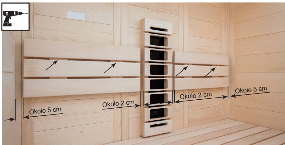
Wiertło 3 mm, 4 szt. śrub 4 x 70 mm
